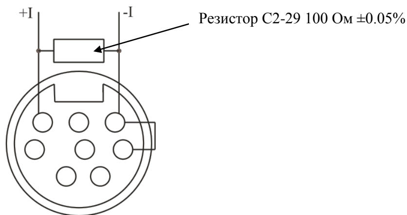
Рисунок 7.2 Входной преобразователь – ПИП с выходным унифицированным
