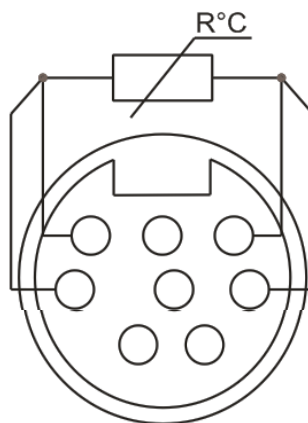
Рисунок 7.3 Входной преобразователь – термопреобразователь сопротивления
